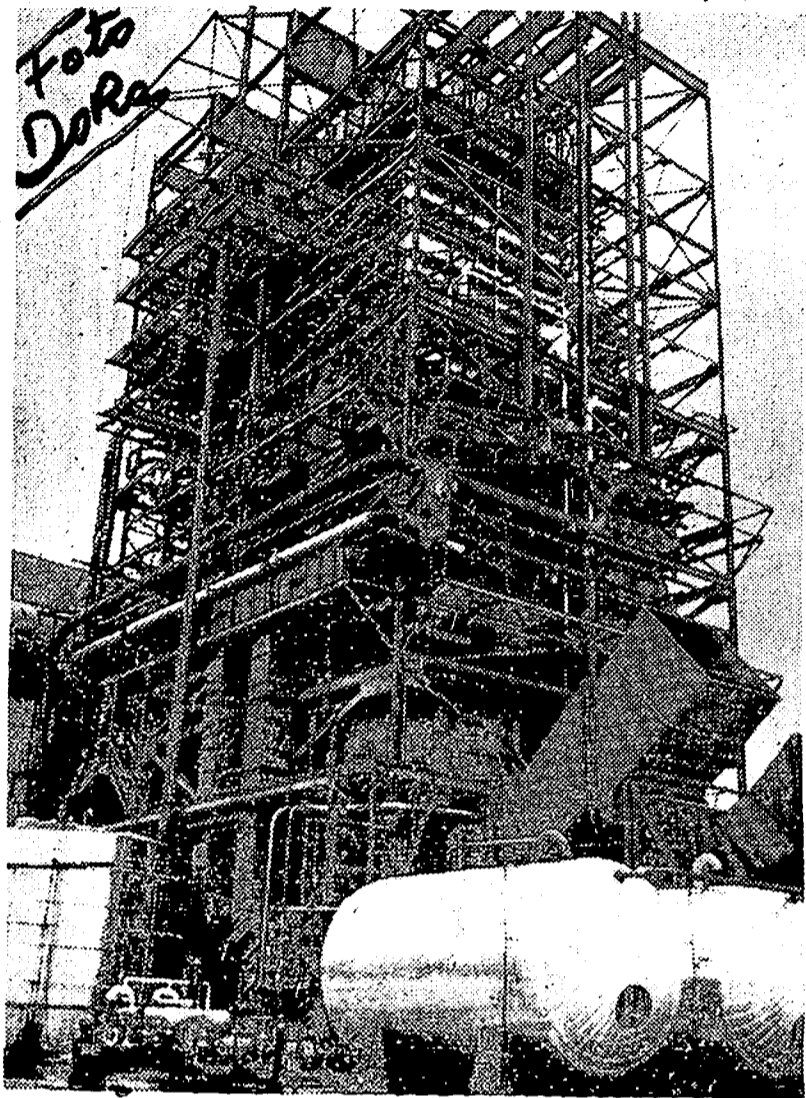
Esta es la gran torre de 60 metros de la Central Térmica de Puente Mayorga, que como se ve, se encuentra ya en muy avanzada fase de construcción y que ayer fue visitada por el alto personal de la Compañía Sevillana de Electricidad.—
